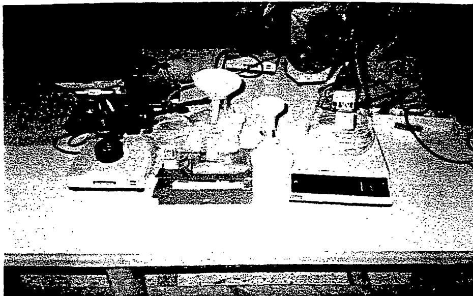
Εικ.14. Τα αντικείμενα και εργαλεία που χρησιμοποιήσαμε. Κωνικές, αλατόμετρο, στερεοσκόπιο, ζυγαριά, χωνιά κ.τ.λ.
