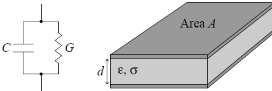
Εικ.1.4 Πυκνωτής
