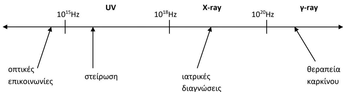
Εικ.1.5 Περιοχή ακτίνων UV, X και γ
