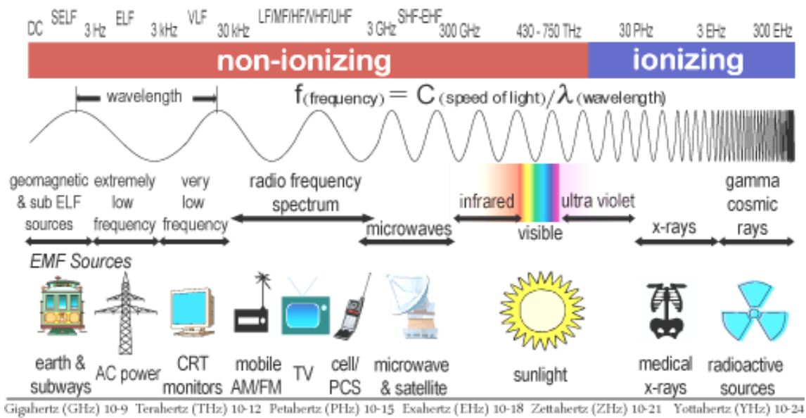
Εικ.1.3 Διαχωρισμός ιοντίζουσας και μη ακτινοβολίας σε σχέση με το μήκος κύματος και την συχνότητα
