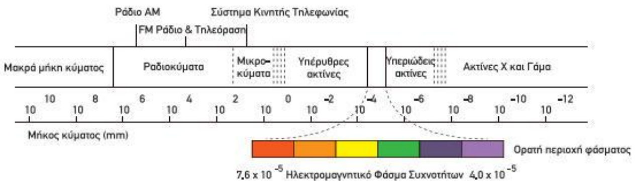
Εικ.1.2 Το ηλεκτρομαγνητικό φάσμα
