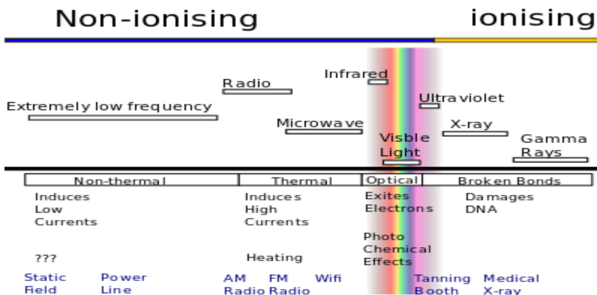
Εικ. 2.2 Σχηματικό φάσμα ιοντίζουσας και μη ιοντίζουσας ακτινοβολίας.
