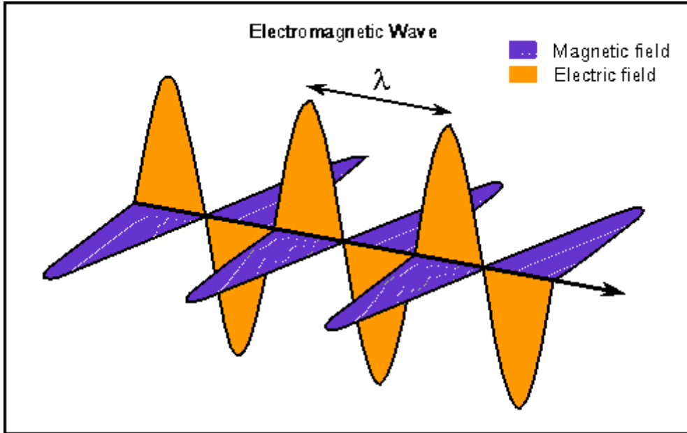
Εικ.1.1 Ηλεκτρομαγνητικό κύμα
