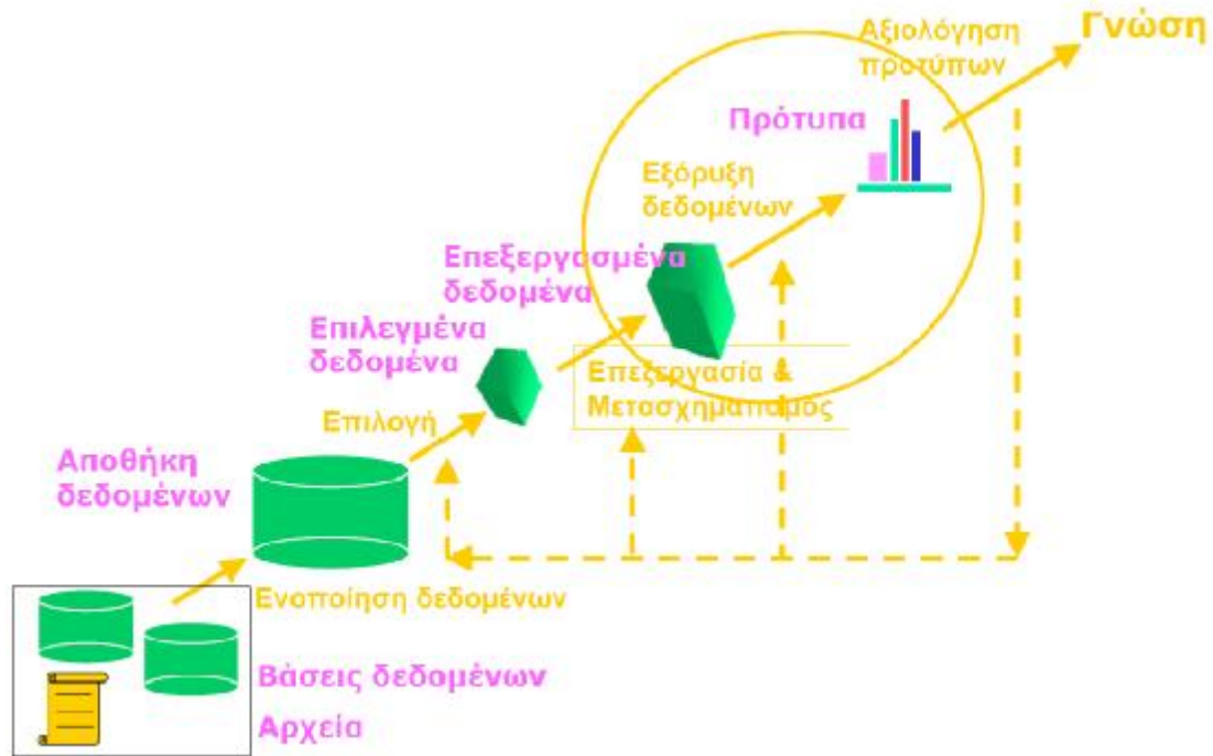
Εικόνα 1: Διαδικασία Ανεύρεσης Γνώσης
