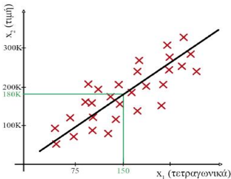
Εικόνα 5: Γραμμική Παλινδρόμηση
