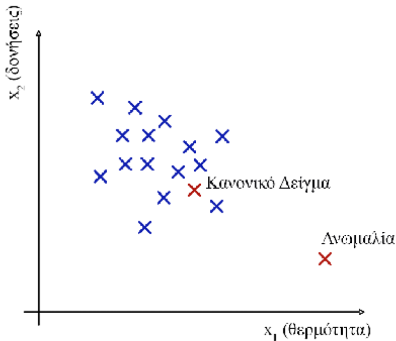
Εικόνα 6: Ανίχνευση Ανωμαλιών
