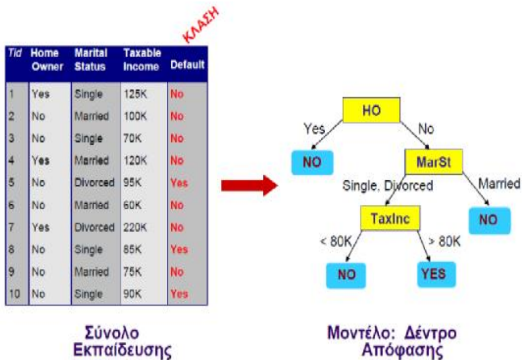
Εικόνα 2: Δένδρα Απόφασης
