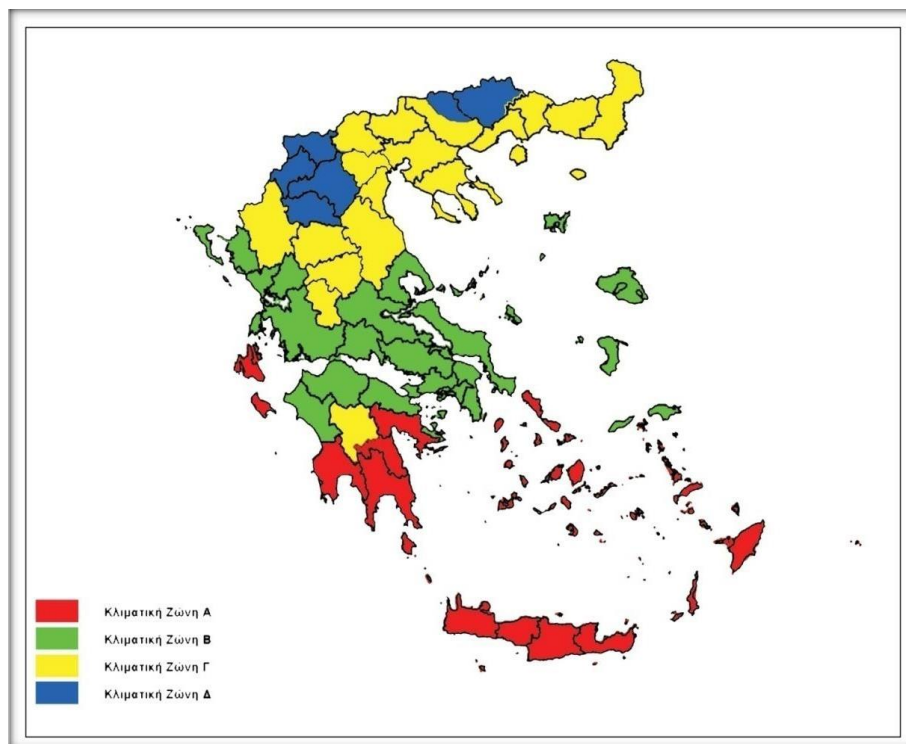
Εικόνα 1.1.: Σχηματική Απεικόνιση κλιματικών ζωνών ελληνικής επικράτειας
